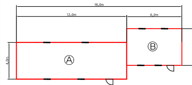
제작 계획 배치도 - 2
